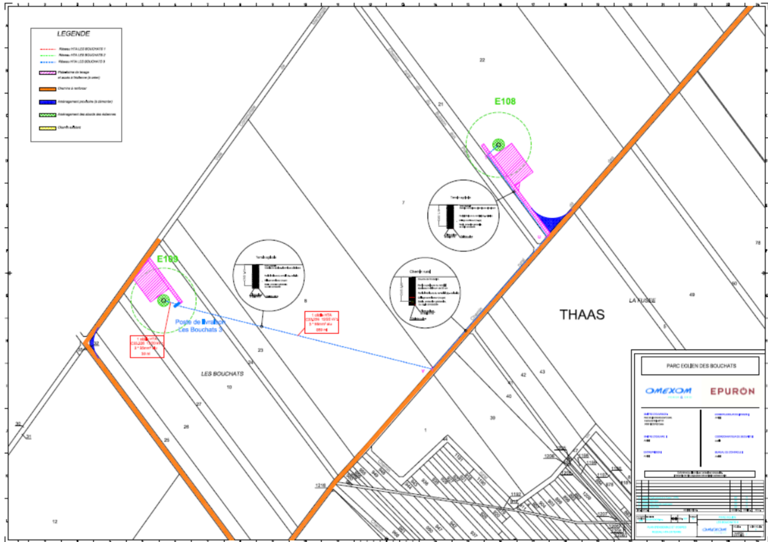
Carte 16 : Plan d'ensemble et coupes - Réseau HTA enterré (source : EPURON, 2015)
