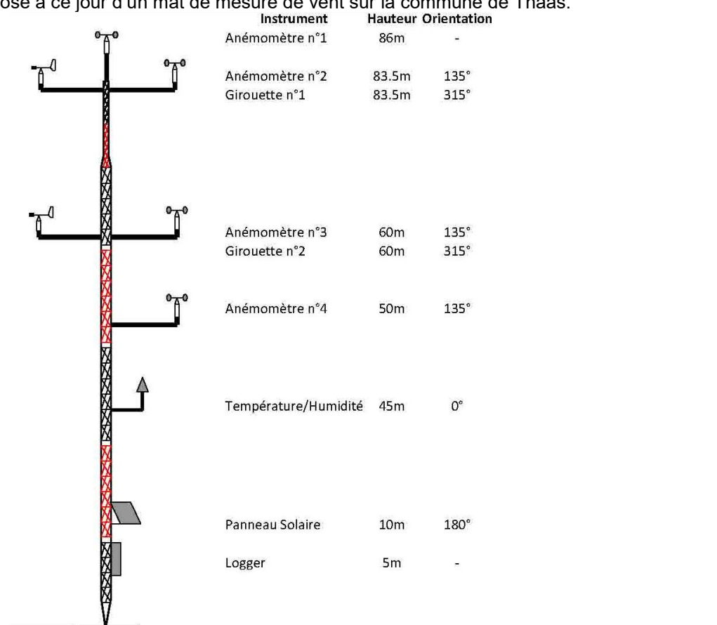
Figure 4 : Illustration du mât de mesure de vent (source : EPURON, 2015)
